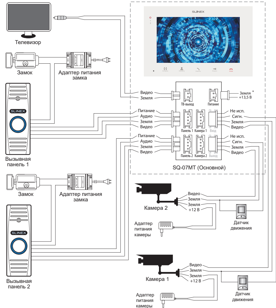
Схема 1. Подключение вызывных панелей, камер и телевизора к домофону SQ-07MT
